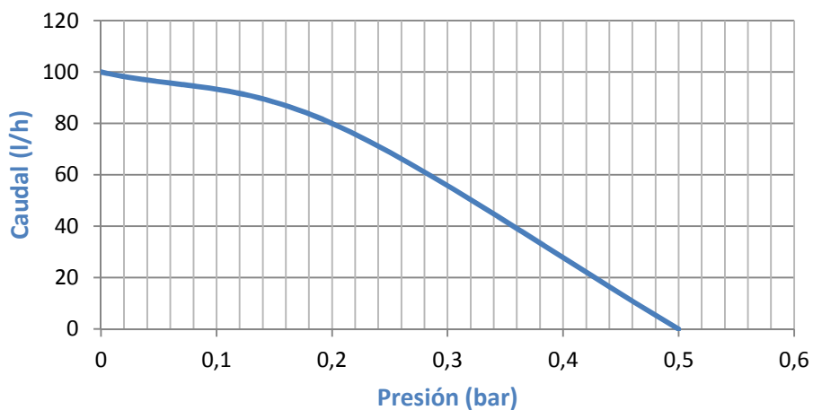
Curva 100/00
