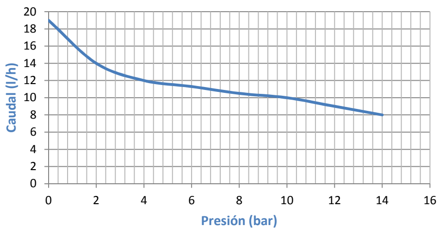
Curva 08/14
